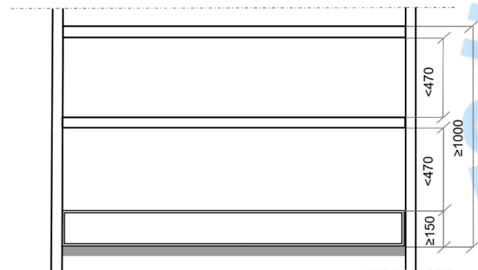
Figura 7.3.2-9: Piccoli trabattelli - Dimensione della protezione laterale
