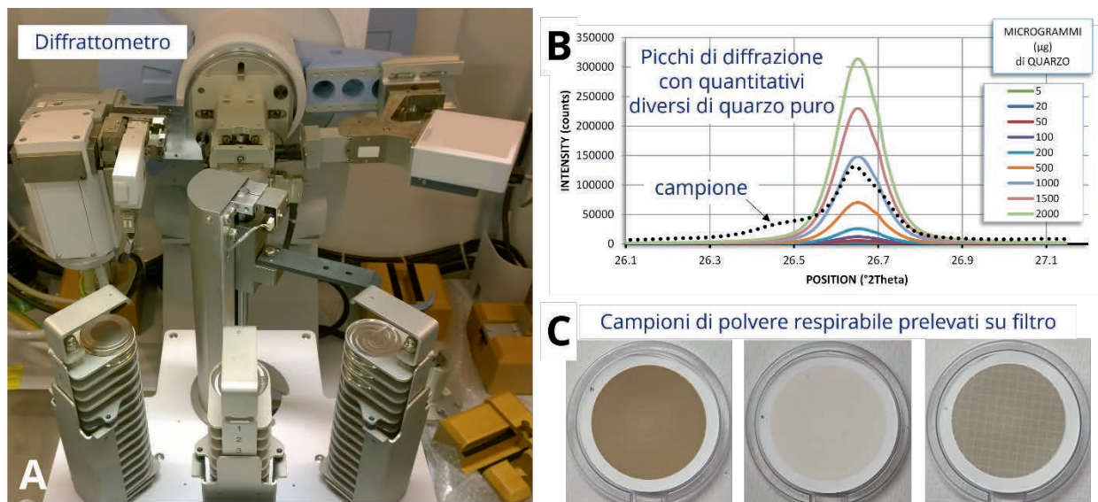
Figura 5. A) Analisi di laboratorio per la determinazione della massa di quarzo sul filtro di campionamento, utilizzando la tecnica della diffrazione dei raggi X. B) Il picco di diffrazione del quarzo è confrontato con quelli ottenuti su filtri di riferimento caricati con quantitativi noti di polvere di quarzo respirabile puro. C) Campioni di polvere respirabile prelevati su filtri in pvc.
